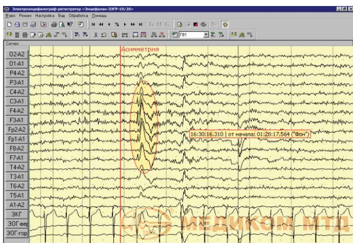
Рис. 4. Пациент У, 21 год. Изолированный комплекс «спайк-медленная волна»
