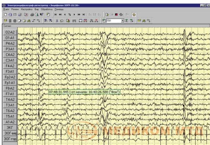
Рис. 5. Пациент У., 21 год. Фрагмент ЭЭГ в утренние часы, через 16 часов после начала записи (компрессированный анализ, экранное время - 40 секунд), периодизация пароксизмальной активности
