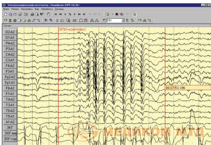
Рис. 3. Пациент У., 21 год. Самый длительный коррелят абсанса обнаружен по дороге домой через 1 час 15 минут после начала записи
